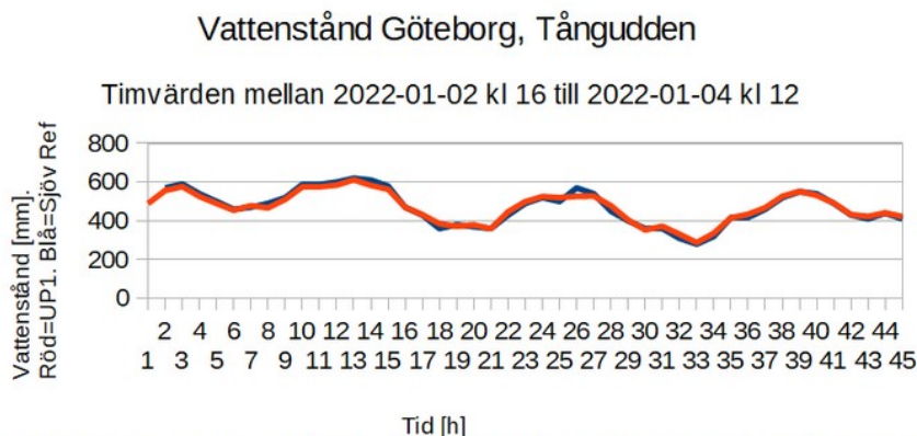
Figur ovan visar att UP1 korrelerar väl med Sjöfartverkets referensstation. UP1 var här ställd att ta 101 'burst mätningar' över en 10-sekunders period för varje genererat mätvärde. UP1 och Sjöfartverkets referensstation var placerade på ett avstånd om ca 400 m.
